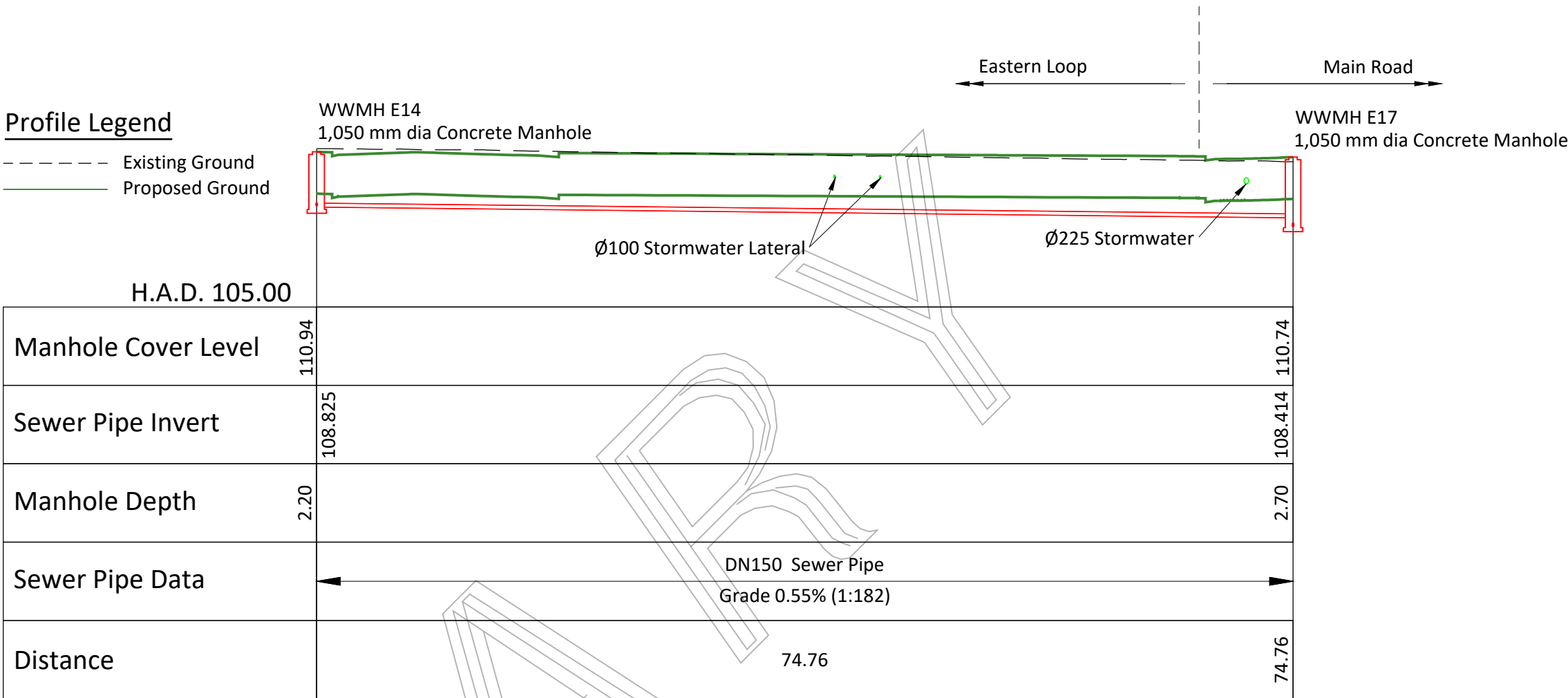
Longsection: WWMH E14 to WWMH E17
